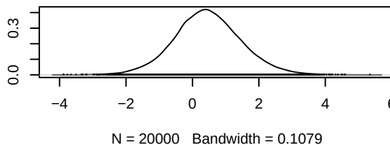
Density of d.Erlotinib.Erlotinib_antiangi
