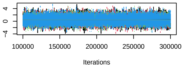
Trace of d.Erlotinib.Erlotinib_antiangi
