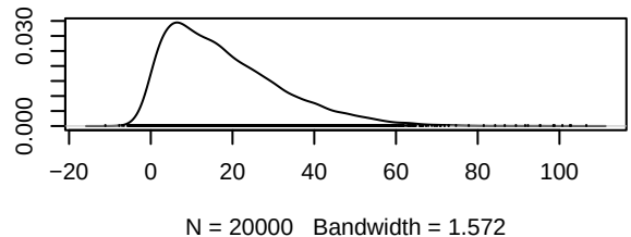
Density of d.Gefitinib.Gefitinib_PARPi
